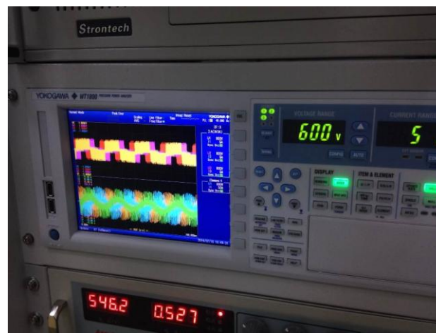
三相电压电流波形显示
